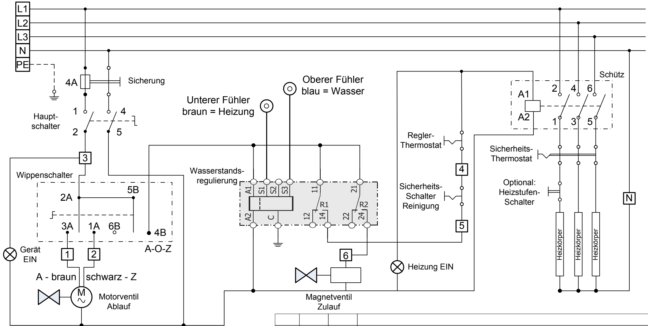
Detail Wasserstandsregulierung
