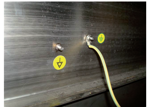
Bild: Anschluss Potentialausgleich
